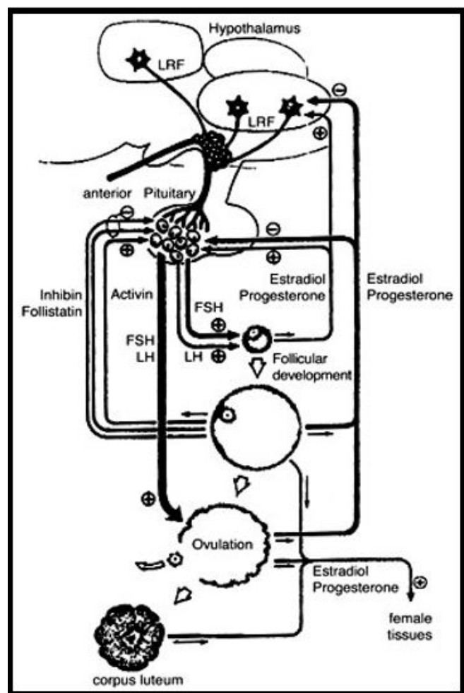
Figura 5: Eventos hormonales del trastorno disfórico premenstrual.
